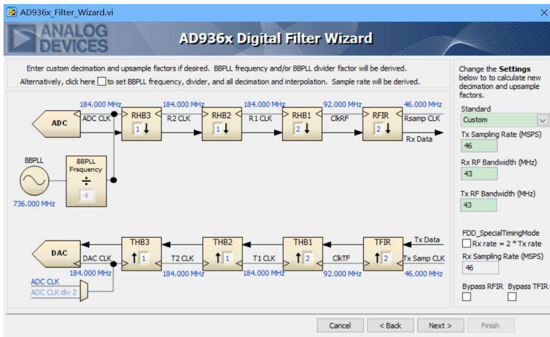
Рис. 1. Интерфейс настройки фильтров в программе AD936X Evaluation Software
