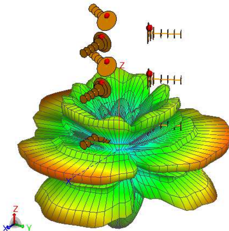
Рис. 1. Модель антенной решетки с трехмерной диаграммой направленности
